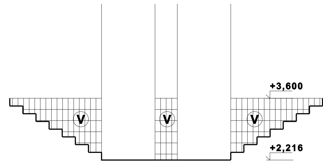
SECTION E1-E1
